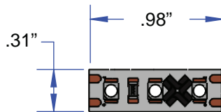
IP65 Flexi-Tape w/120 LEDs per meter (set)
