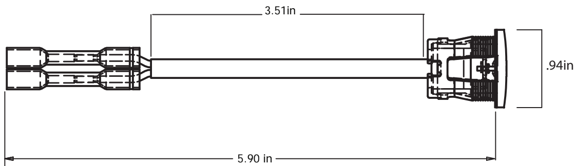
#480034 without grommet
